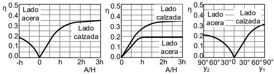
Curvas del factor de utilización
