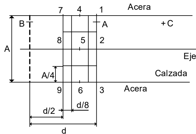
Distribución de puntos en una disposición unilateral
