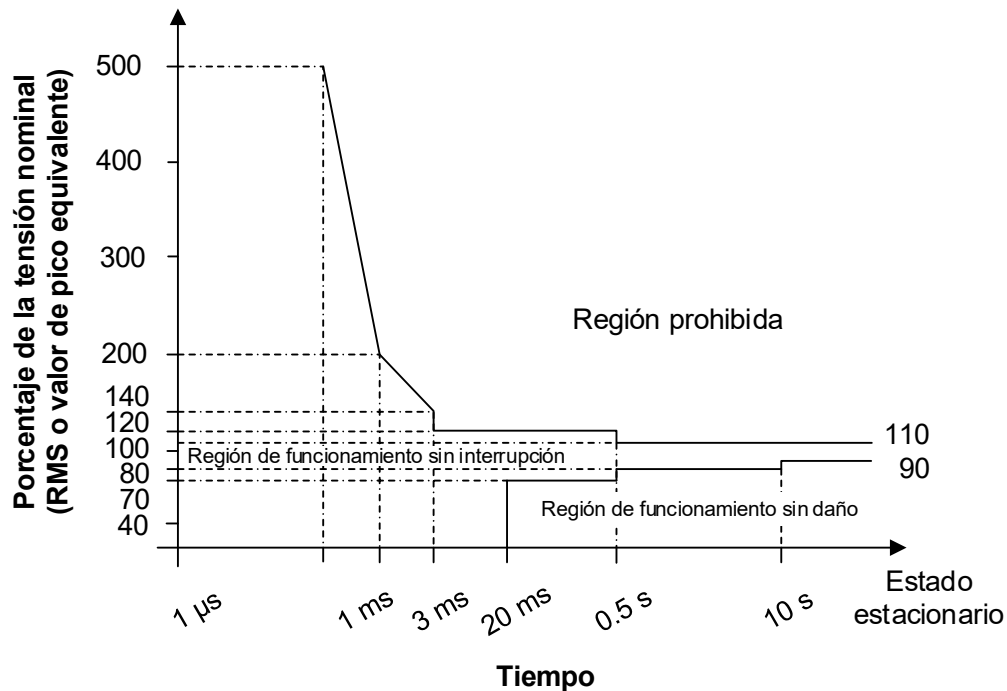
Figura 3.1.1.A. Curva ITIC o ITI (desarrollada por el Consejo Industrial de Tecnología de la Información, en inglés Information Technology Industry Council)
